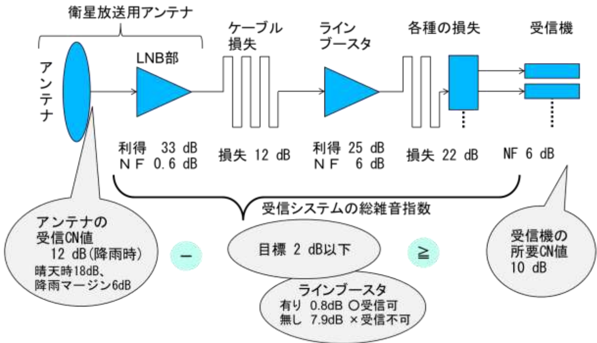
図 3-6 受信システムの設計例
