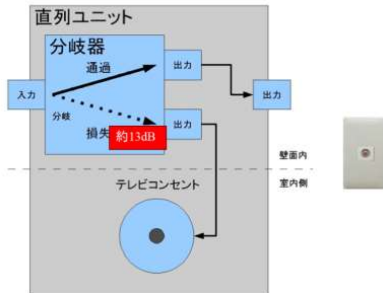
図 3-23 直列ユニット
