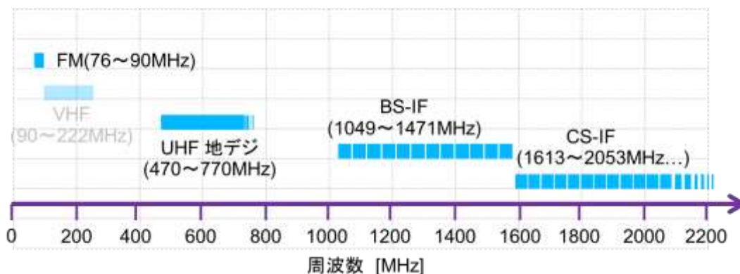
図 2-3 放送周波数
