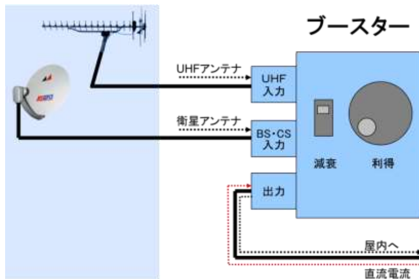
図 3-26 ブースターの混合機能
