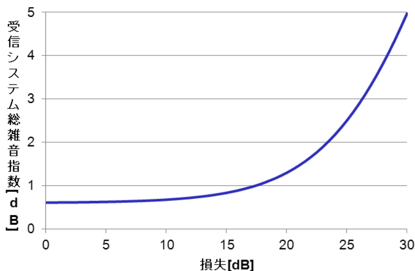
図 3-5 アンテナ以降の損失と受信システム総雑音指数(総 NF)の計算例
