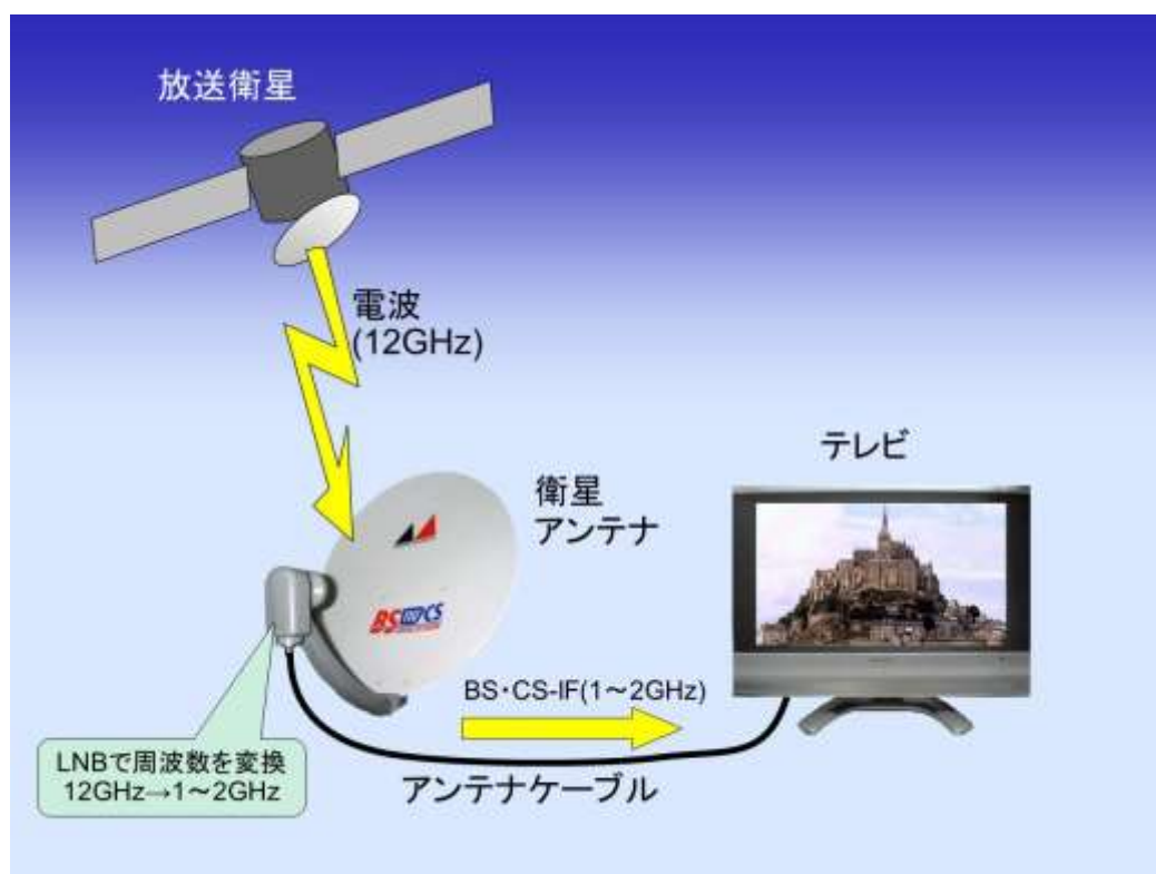
図 2-1 LNB の役割
