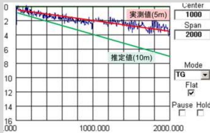
図 2-4 S-4C-FB ケーブルの周波数特性
