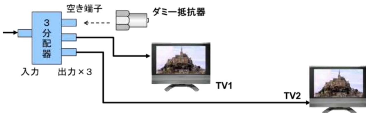
図 3-14 分配器の空き端子にはダミー抵抗器を取り付ける
