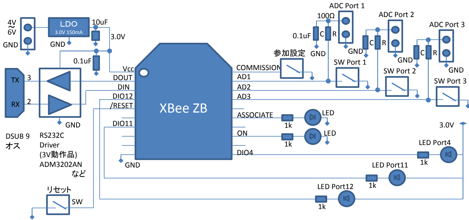
Coordinator/End Device共用XBee基板回路図
